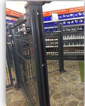
U-Leiste montiert
